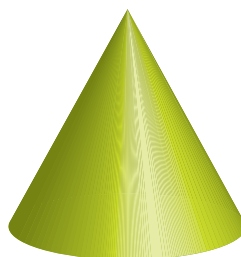
Cone
